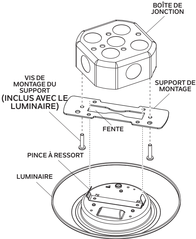
Fig. 1 INSTALLATION SUR UNE BOÎTE DE JONCTION STANDARD
