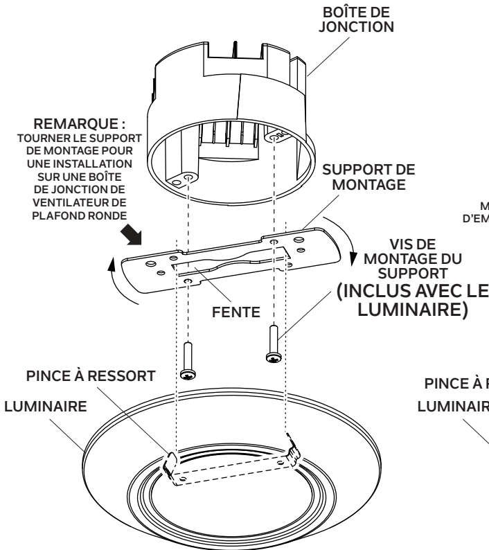
Fig. 2 INSTALLATION SUR LA BOÎTE DE JONCTION DU VENTILATEUR DE PLAFOND RONDE
