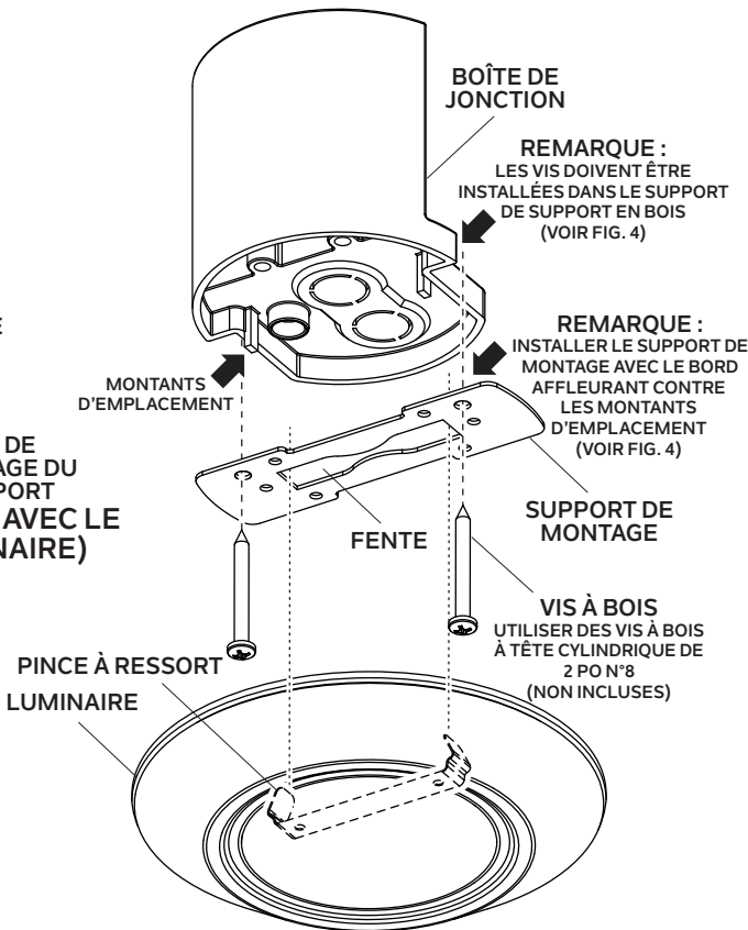
Fig. 3 INSTALLATION SUR LA BOÎTE DE JONCTION DU VENTILATEUR DE PLAFOND EN FORME DE L
