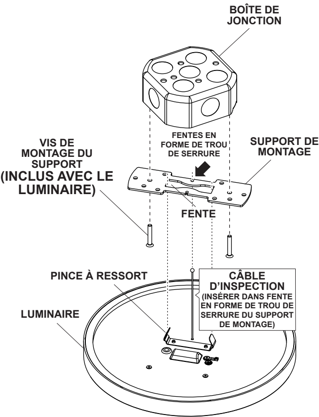
Fig. 1 INSTALLATION SUR UNE BOÎTE DE JONCTION STANDARD
