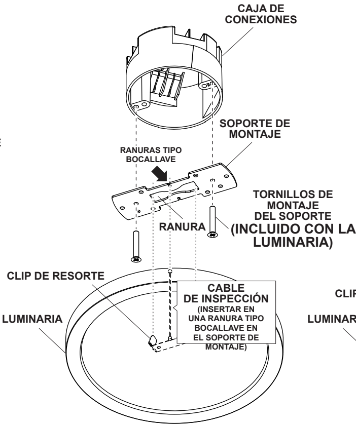
Fig. 2 INSTALACIÓN EN CAJA DE CONEXIONES DE VENTILADOR DE TECHO REDONDA
