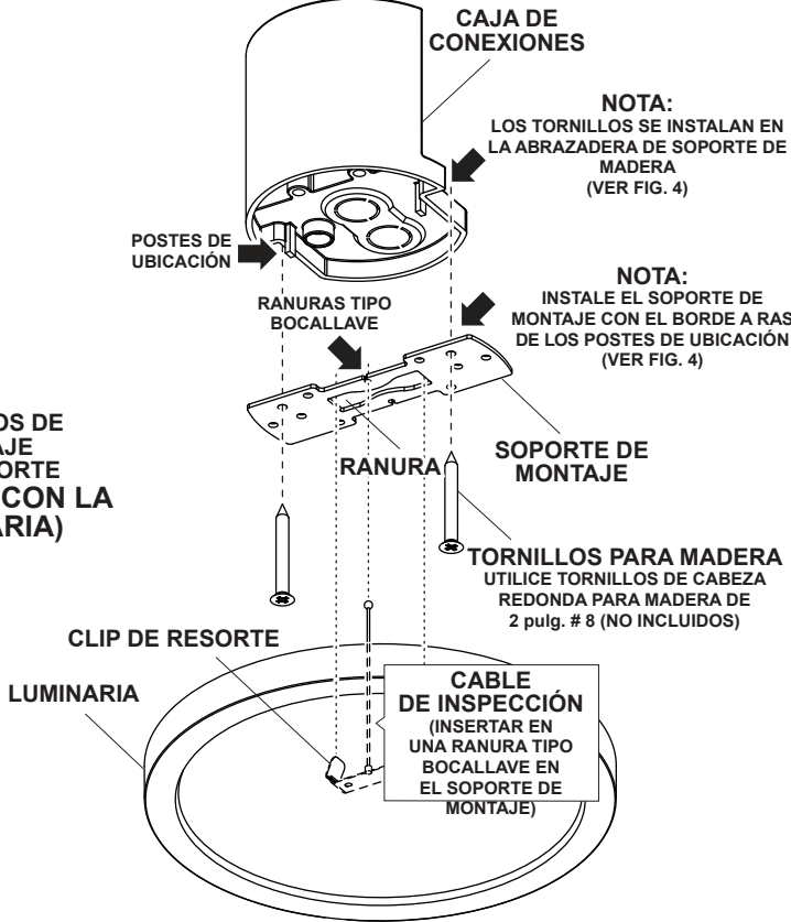
Fig. 3 INSTALACIÓN EN CAJA DE CONEXIONES DE VENTILADOR DE TECHO EN FORMA DE L
