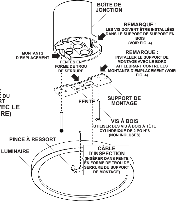
Fig. 3 INSTALLATION SUR LA BOÎTE DE JONCTION DU VENTILATEUR DE PLAFOND EN FORME DE L
